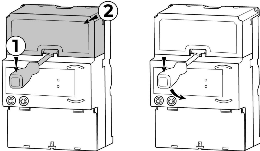
Рисунок 6.4 – Доступ к сменному модулю связи
