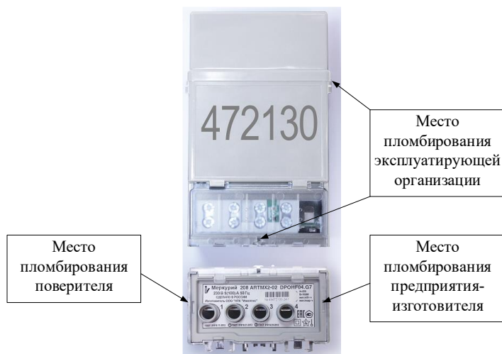
Рисунок 3.3 – Общий вид счетчиков «Меркурий 208» с индексами «М» и «Х» с указанием мест пломбирования и нанесения знака поверки
