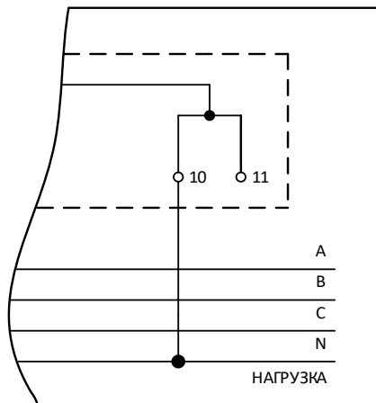
Рисунок Б.9 – Схема с подключением только одного проводника нейтрали
