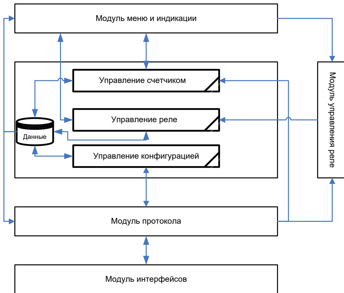
Рисунок 2.5 – Алгоритм индикации и управления
