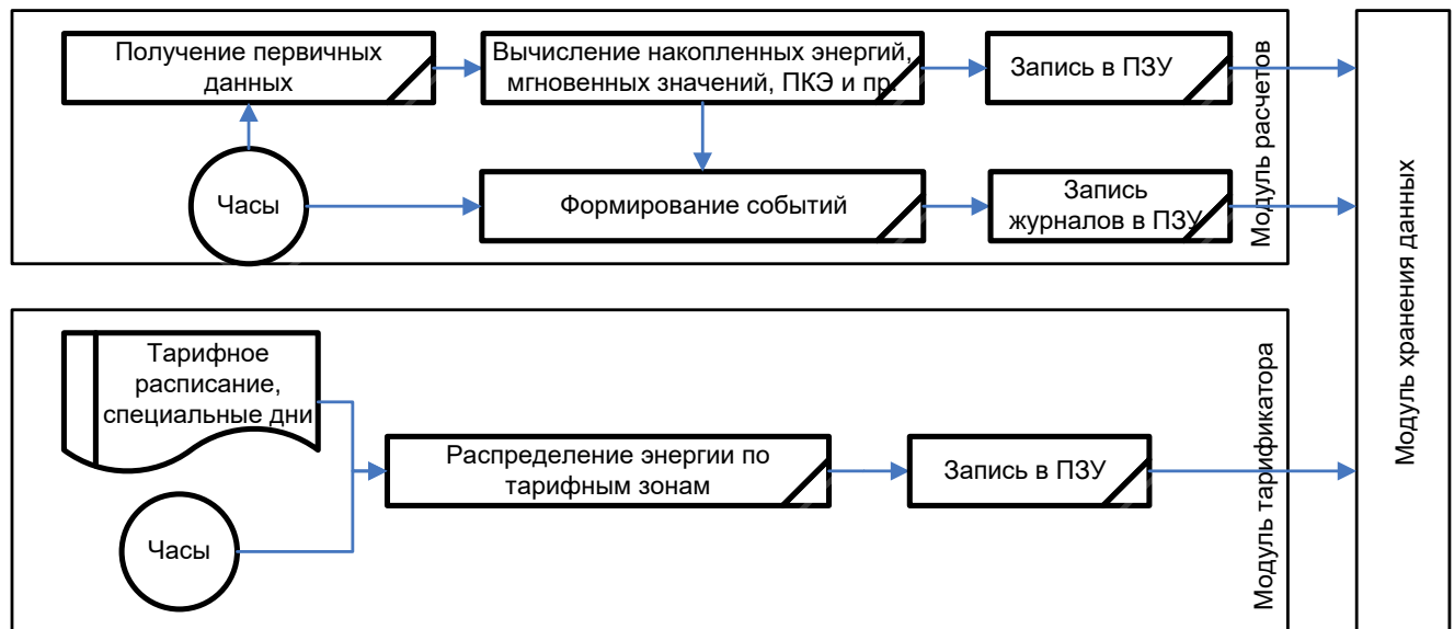
Рисунок 2.4 – Алгоритм сохранения данных
