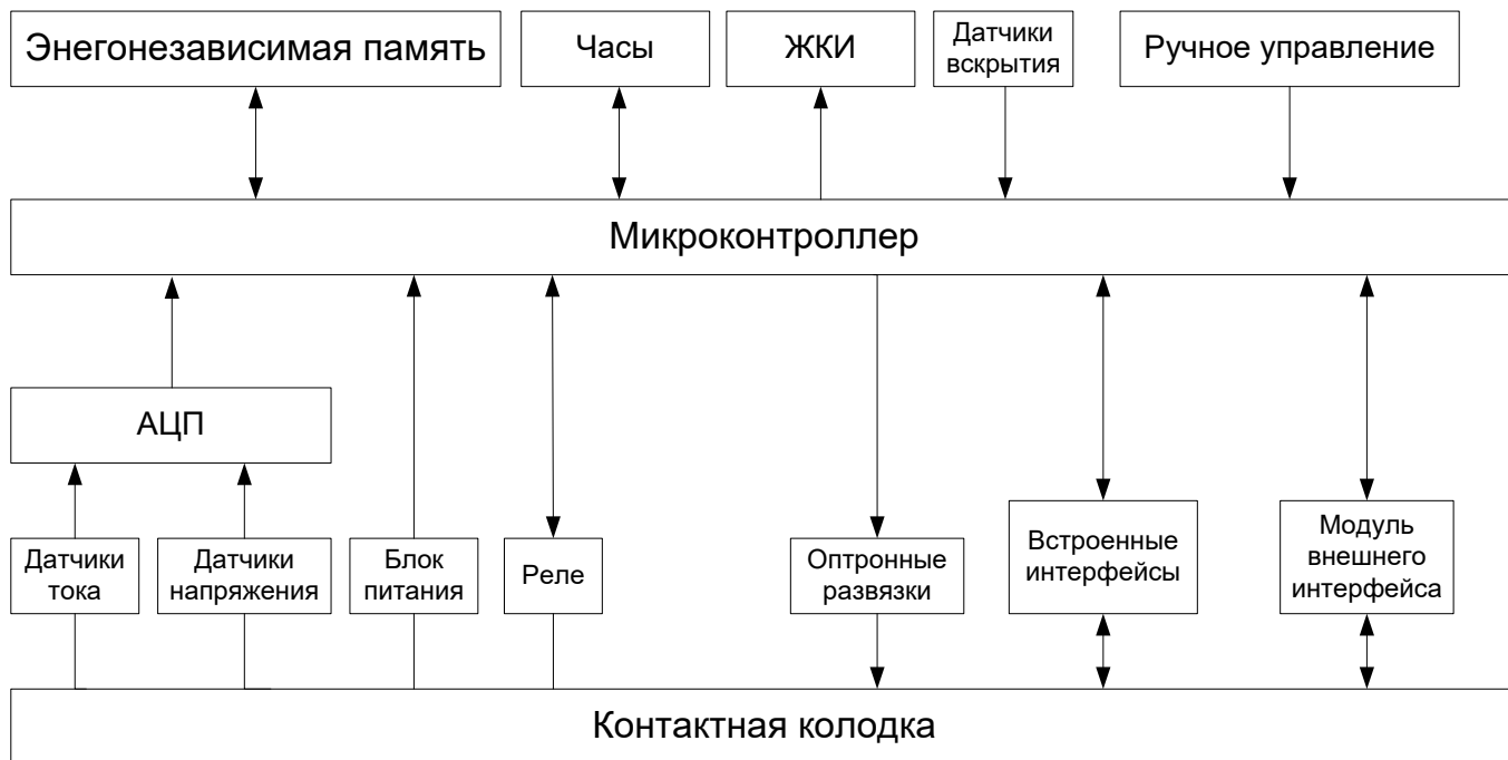
Рисунок 2.1 – Структурная схема ПУ и ВПО
