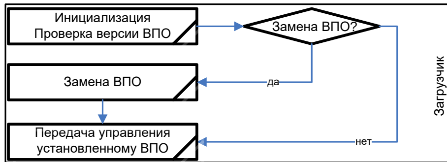
Рисунок 2.3 – Алгоритм работы модуля загрузчика
